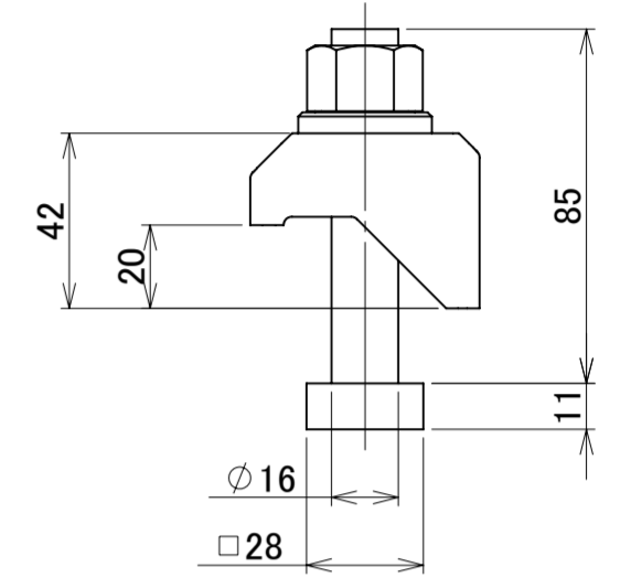
クランプブロック寸法図 4セット付属(ブロック、ボルト、ナット、ワッシャ)
